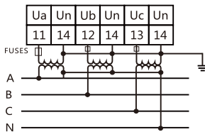
3PT(三相四线3P4L)
