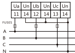
三相四线3P4L
