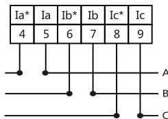
电流直接输入
