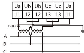
2PT(三相三线3P3L)
