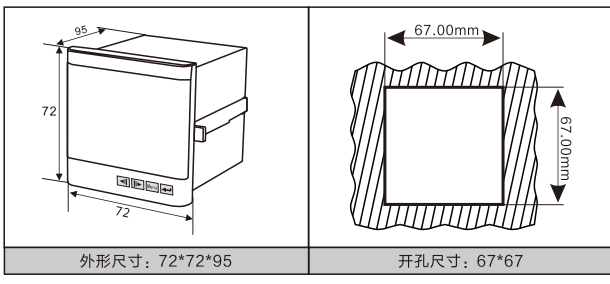
■72方型 (外形尺寸: 72*72*95 mm 开孔尺寸: 67.00*67.00mm)
