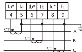
电流经3CT输入
