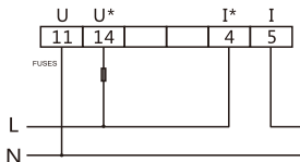
电流直接输入
