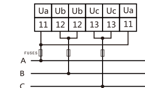
三相三线3P3L
