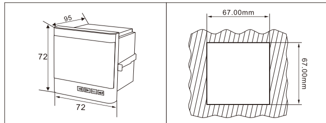
外形尺寸: 72×72×95
